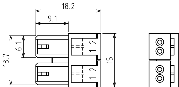
2芯2連分離形ソケット 232D-02S1A2-DA5-FA
