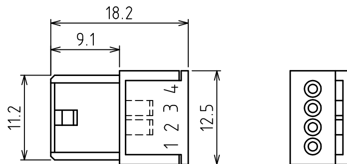
2/4芯分離形ソケット 232D-04S1B-DA5D1(02)-FA
