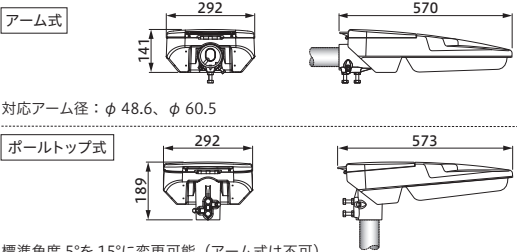
写真は KLE-143S-73L-PT
